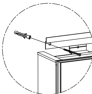
挂片底部贴在镜柜上挂码局部示意图
